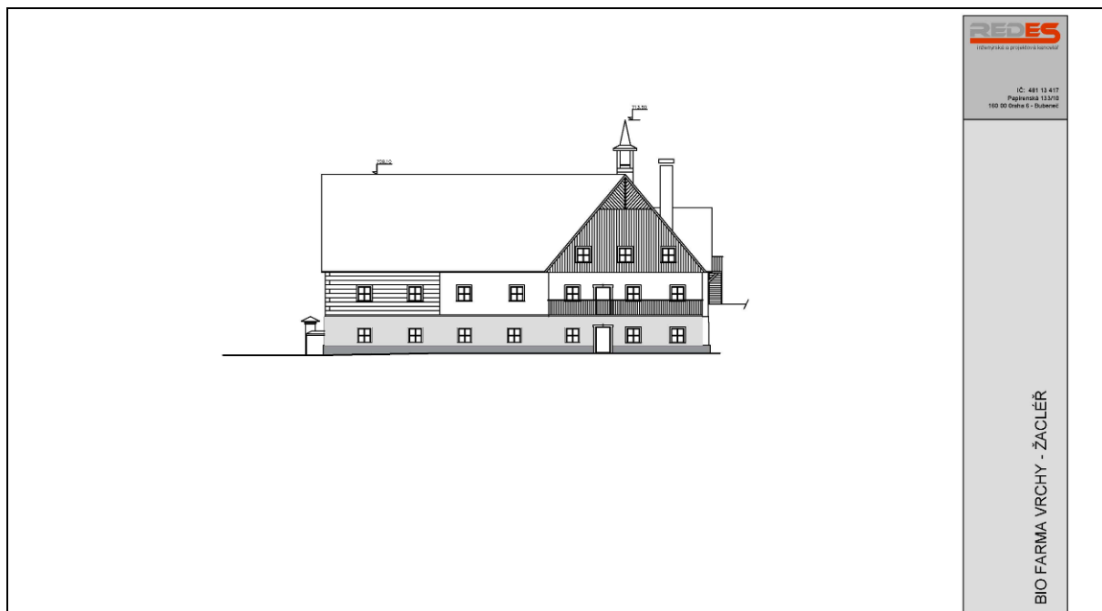
pohled východní
